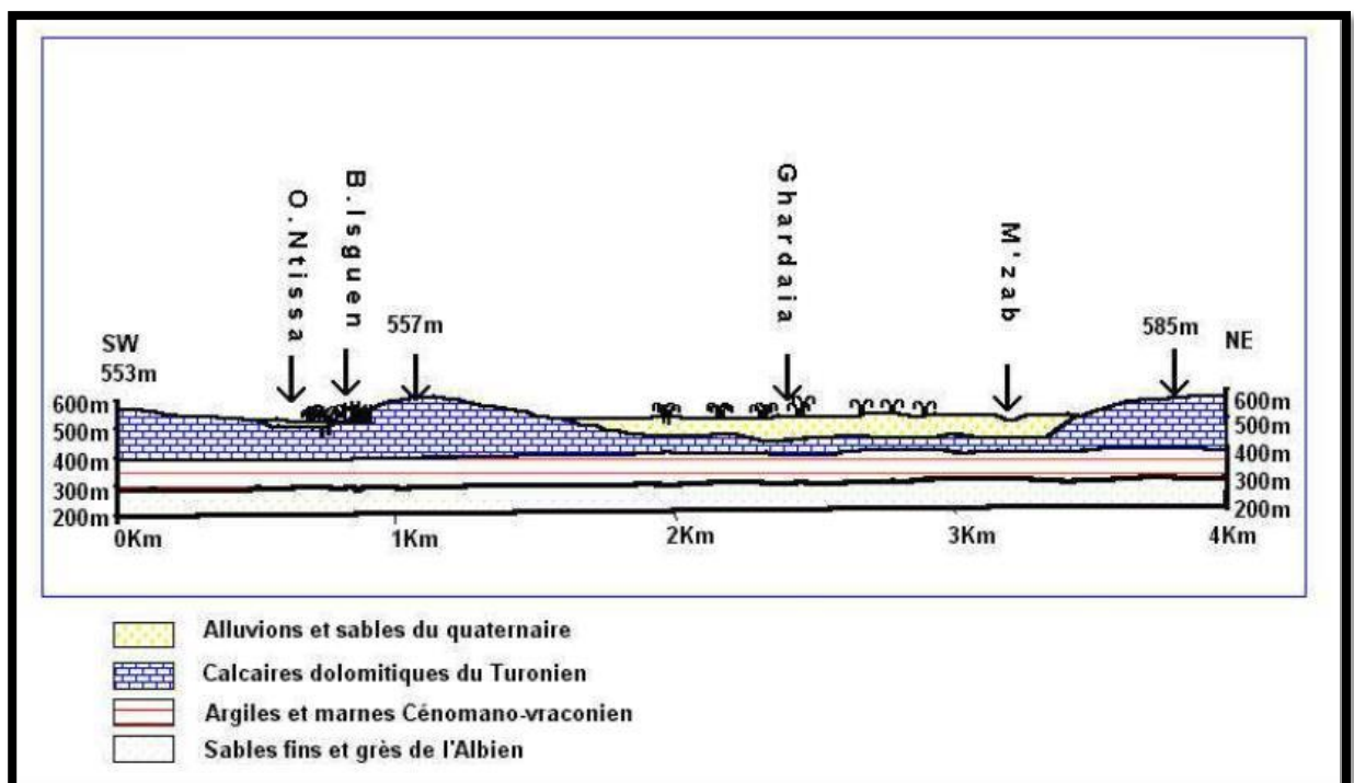
Fig. n° 08 : Coupe géologique schématisée de la région du M'Zab
